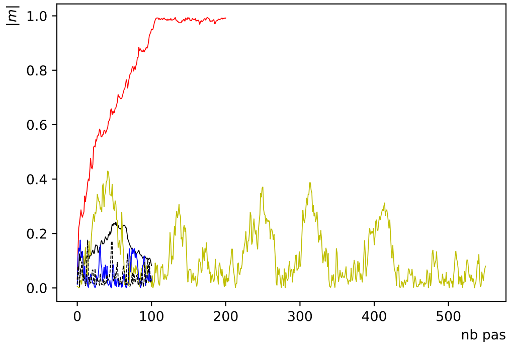
Evolution selon critère Estimation par intervalle,Condition Initiale aléatoire de taille L=32
